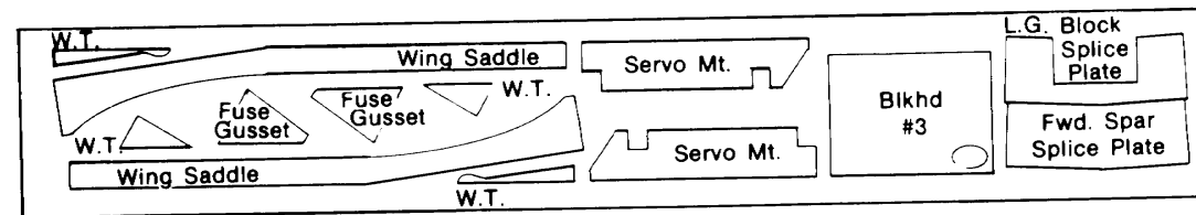
D.C. #4 - 1/8 X 3 X 23
